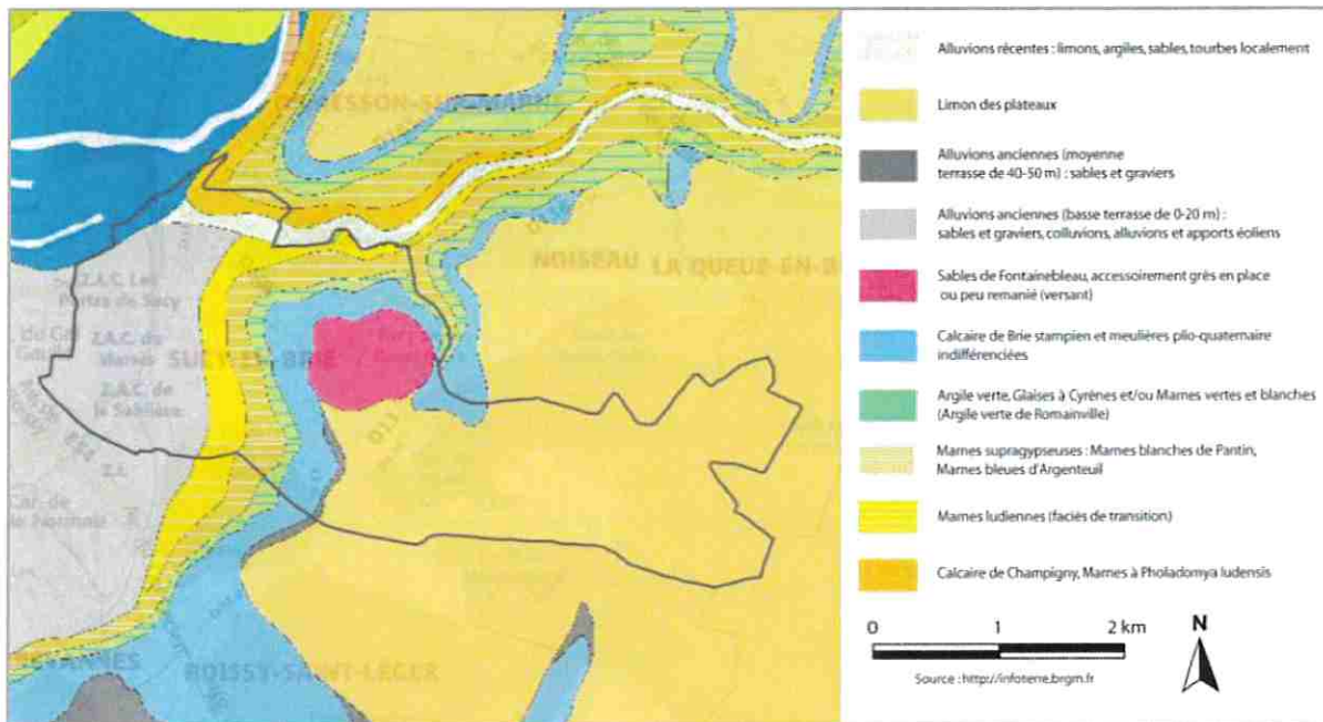
Contexte géologique de Sucey-en-Brie (Source : PLU actuel)
